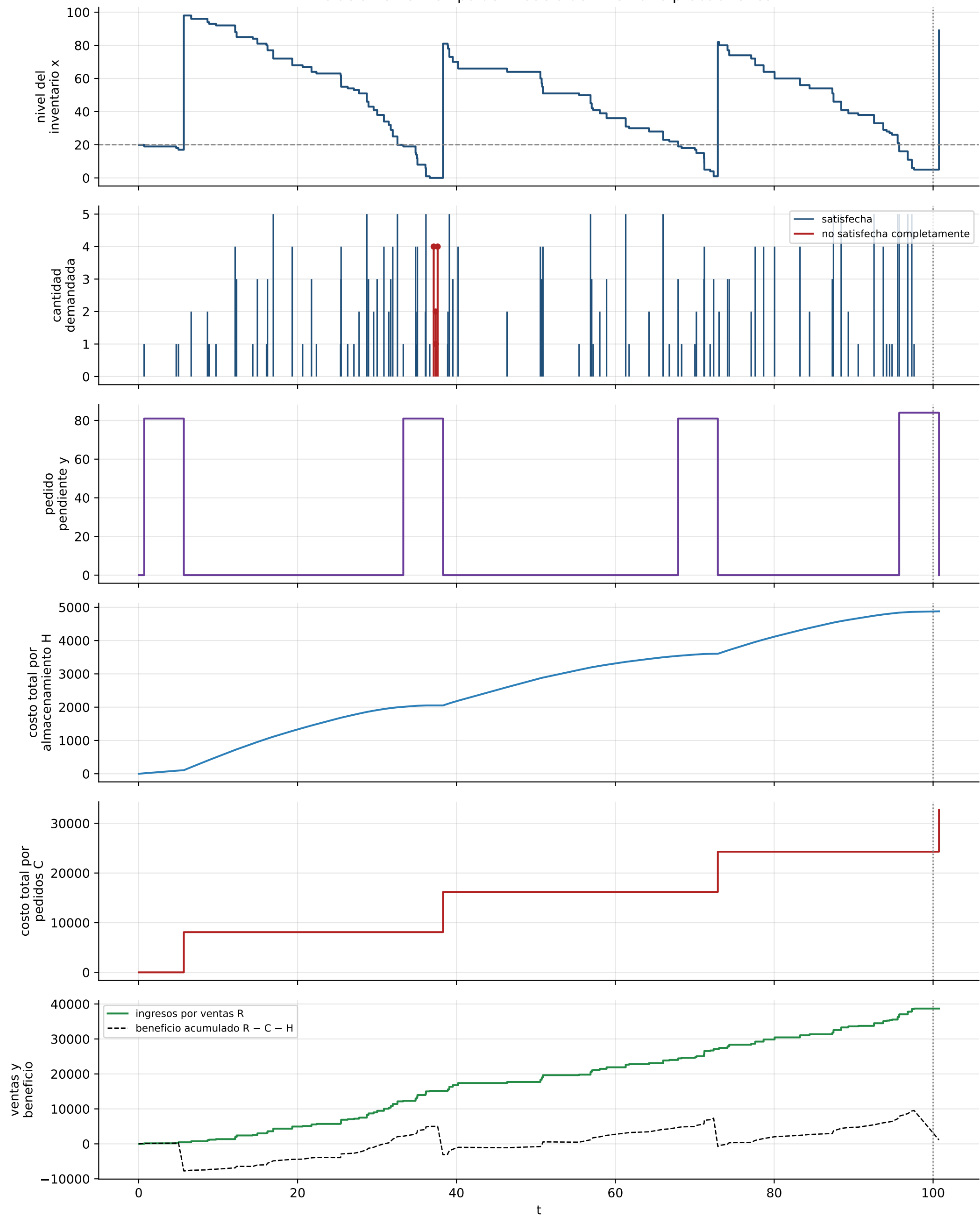
Evolución en el tiempo del modelo de inventario probabilístico
